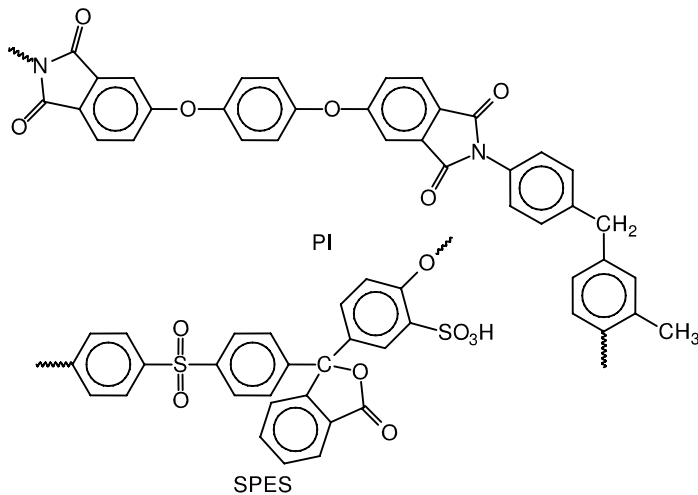
الشكل (11-7): بولي (إيميد) وپولي (إيثر سلفون) المُسلفن 81
